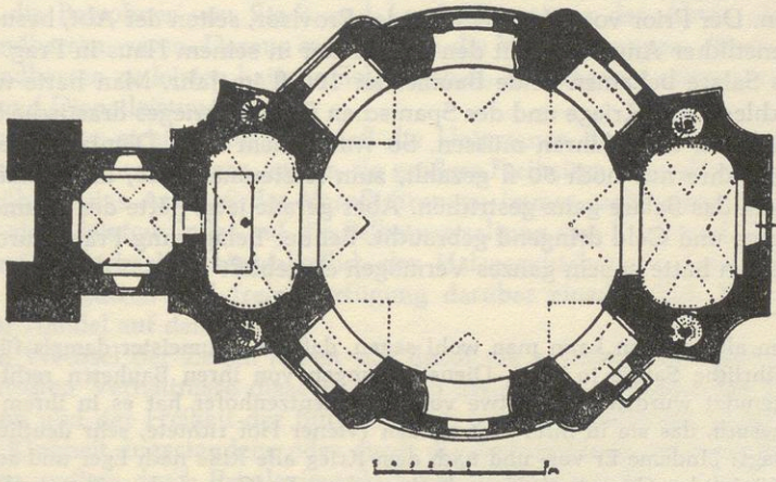
Grundriß der Kirche zu Barzdorf
