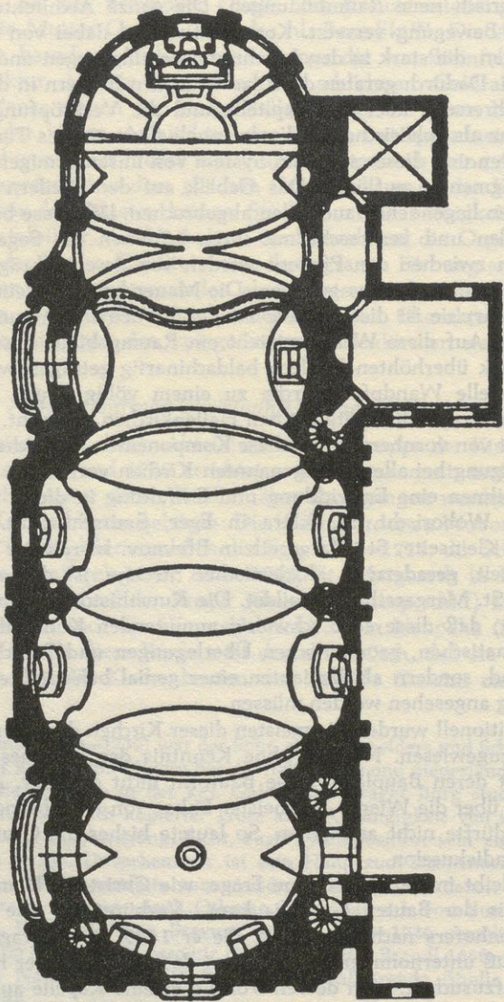
Grundriß der Abteikirche St. Margareth in Břevnov
