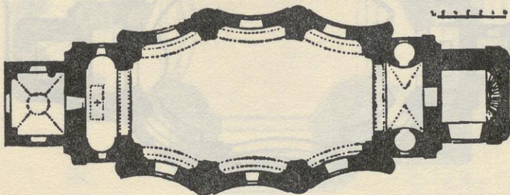
Grundriß der Hermsdorfer Pfarrkirche
