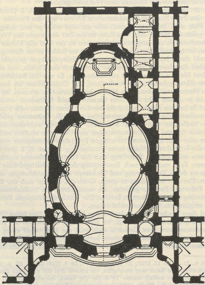
Grundriß der Propsteikirche in Wahlstatt
