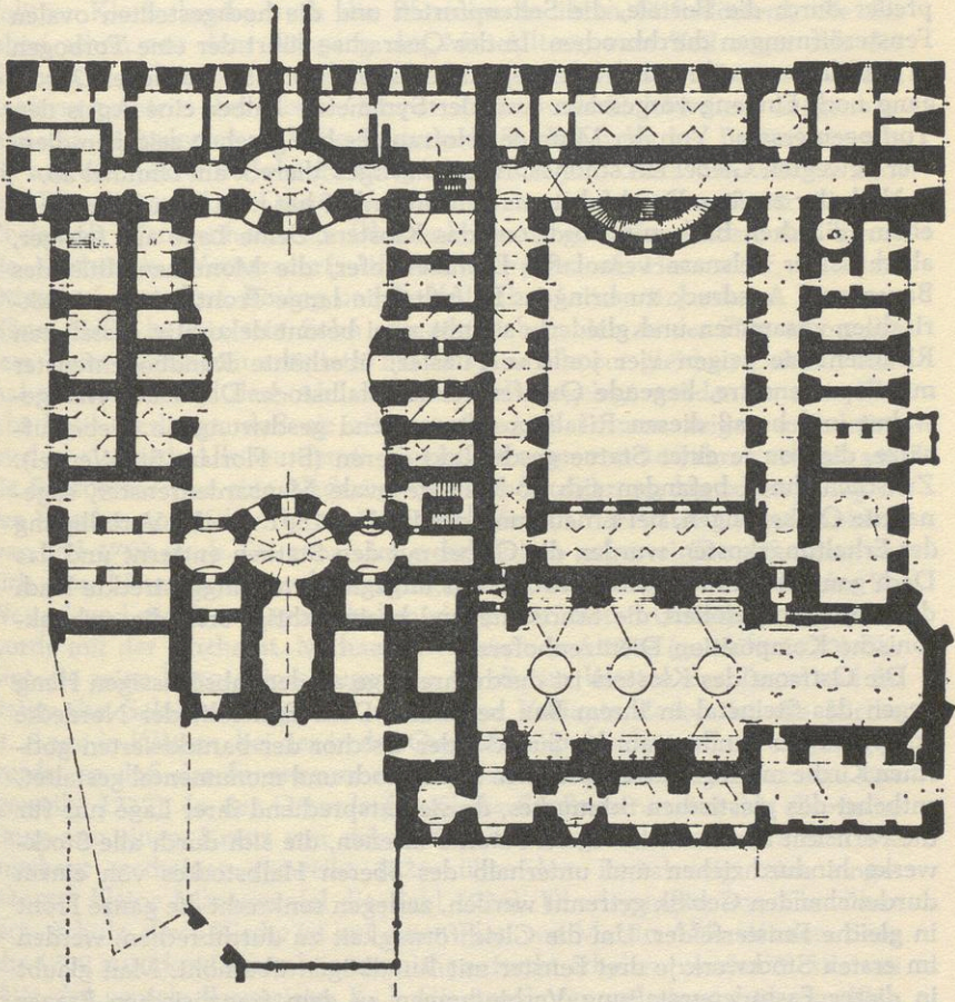
Grundriß des Klosters und der Kirche in Braunau
