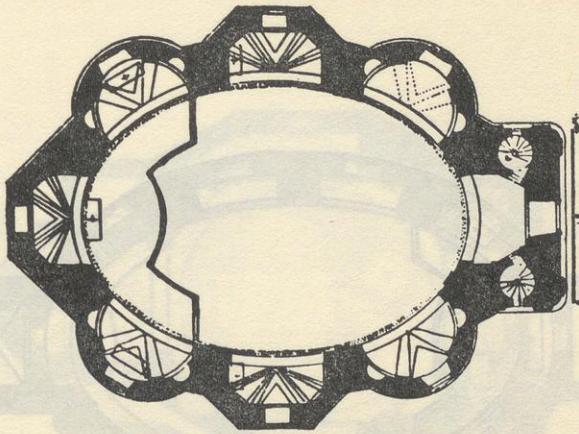
Grundriß der Kirche in Ottendorf
