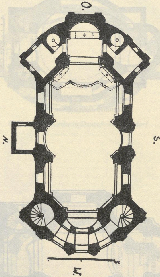
Grundriß der Kirche zu Schönau
