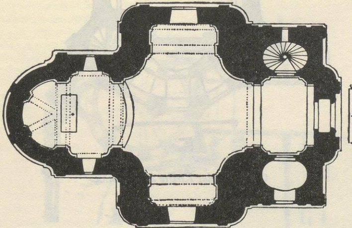
Grundriß der Kirche St. Wenzel in Braunau
