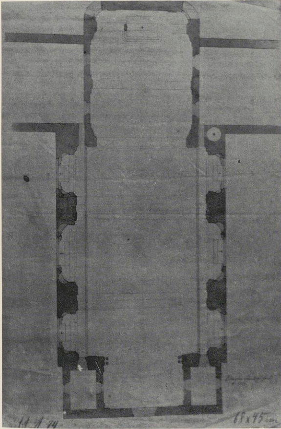
11. P. J. Schaukegl, Plan einer Stiftskirche, 1760, Grundriß
