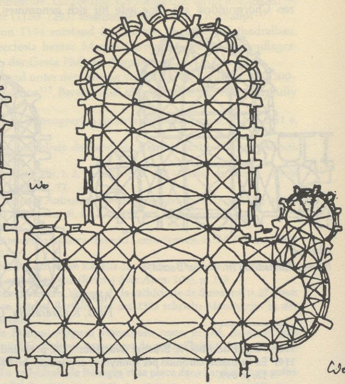
Abb. 19 Soissons, Kathedrale (n. Dehio/Bezold)
