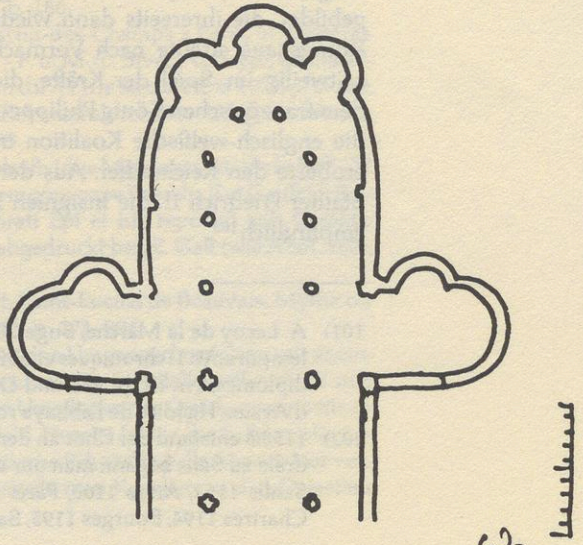
Abb. 11 Aversa, Kathedrale (n. Muscie)
