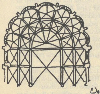
Abb. 12 Saint-Denis, Abteikirche (n. Dehio/Bezold)
