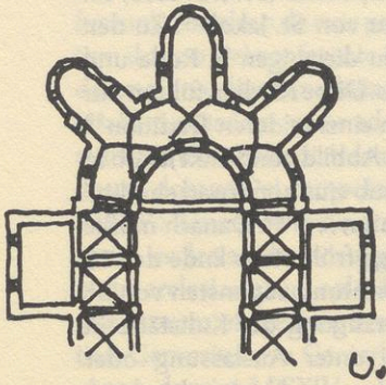
Abb. 5 Angers, Kathedrale (n. Farcy)
