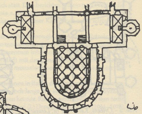
Abb. 7 Hildesheim, St. Michael (n. Beseler/Roggenkamp)
