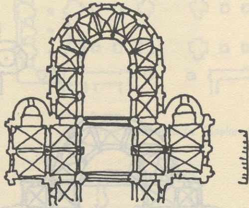
Abb. 3 – Jumièges, Abteikirche (n. Lanfray)
