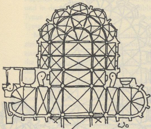
Abb. 14 Noyon, Kathedrale (n. Dehio/Bezold)
