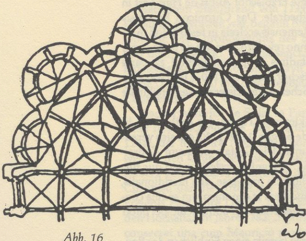
Abb. 16 Chartres, Kathedrale (n. Dehio/Bezold)
