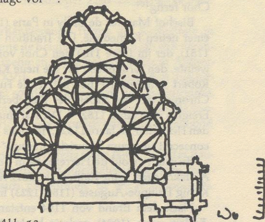
Abb. 13 Paris, St. Martin-des-Champs (n. Dehio/Bezold)
