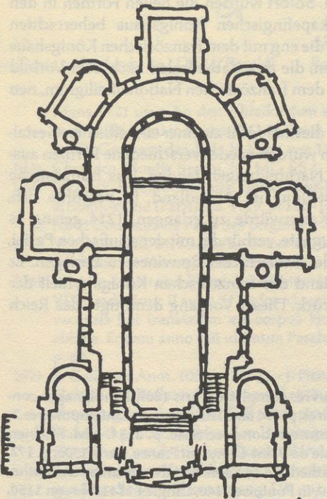
Abb. 10 Canterbury, Kathedrale (n. Bond)
