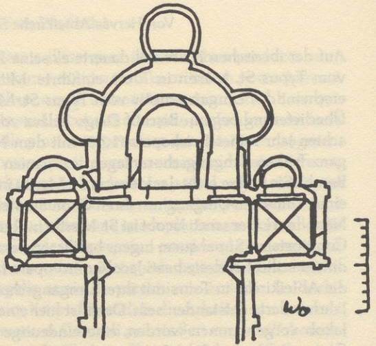
Abb. 4 Chartres, Kathedrale (n. Branner)
