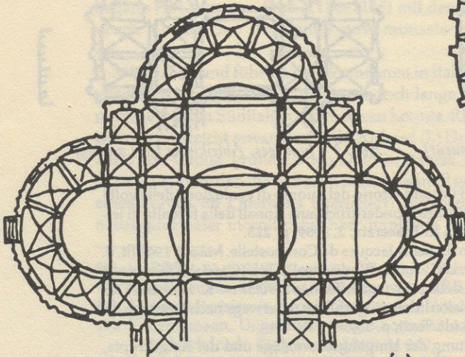
Abb. 6 Köln, St. Maria im Kapitol (n. Dehio/Bezold)
