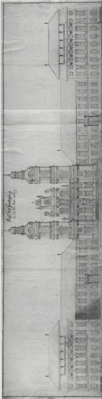
Abb. 4: Johann Lucas von Hildebrandt, erstes Projekt für den Neubau des Stiftes Göttweig, Aufriß, 1719 (Graphische Sammlung, Inv.-Nr. W c 024)
